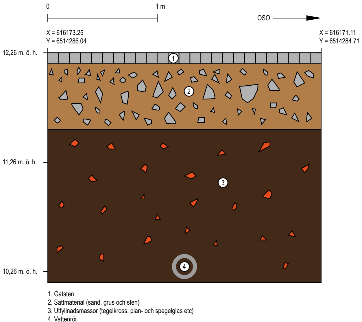
Figur 3. Schaktets södra kortsida i profil. Skala 1:20
